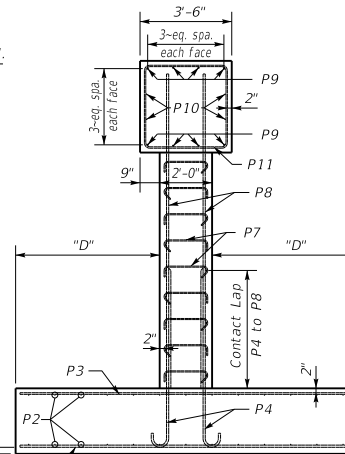
END ELEVATION
